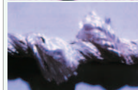
Abb. 7: Schnittverletzung bei einem gedrehten Seil; eine ganze Litze ist durchtrennt
